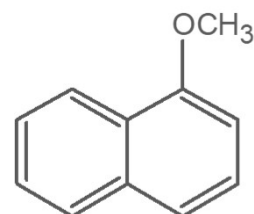
1-METOXYNAPHTALENE
